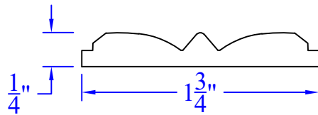
MLDG091 1/4" x 1-3/4"
